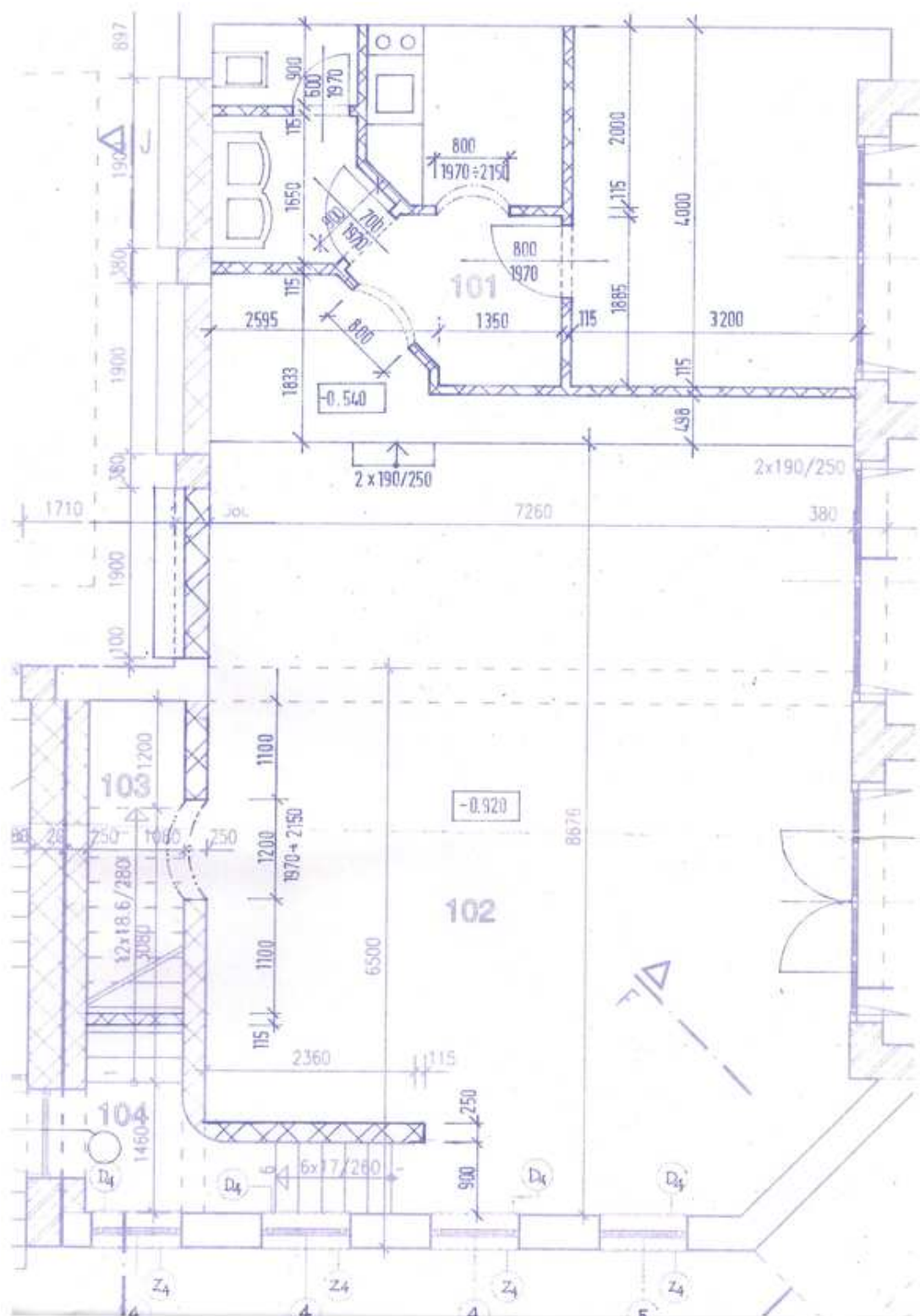
Pôdorys 1. poschodia:
